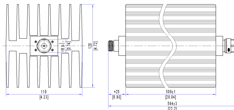
Outline A: Without Fan
